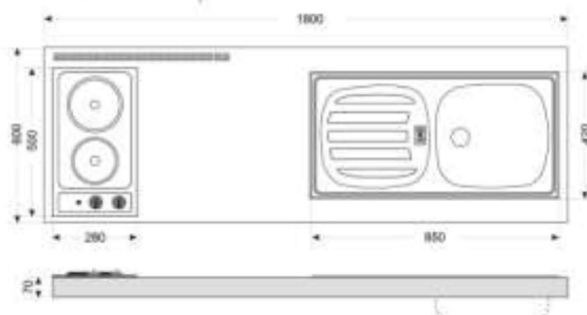
Croquis de la encimera Top 180
