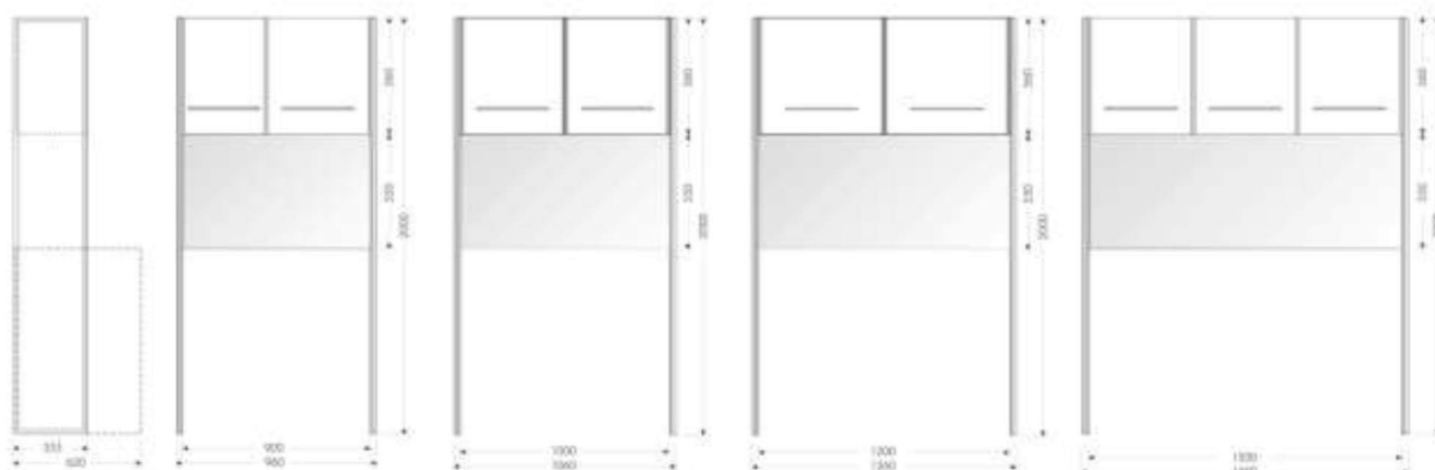
Studioline E Boceto lateral
